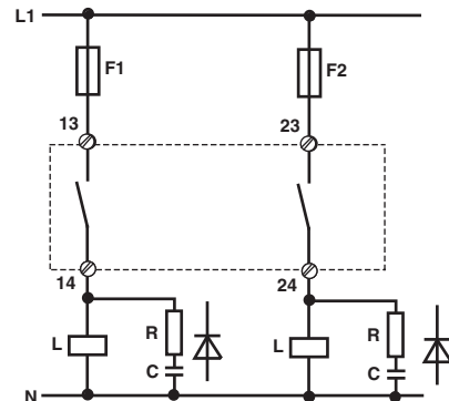
Fig. 4: Funkenlöschung Spark suppression Extinction d'arc
