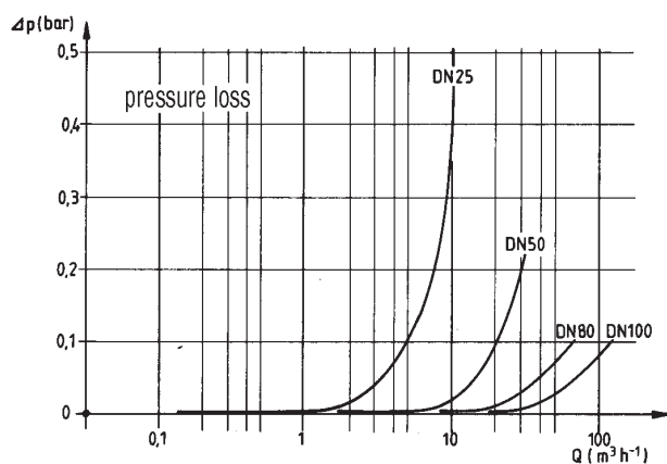
Диаграмма потери давления
