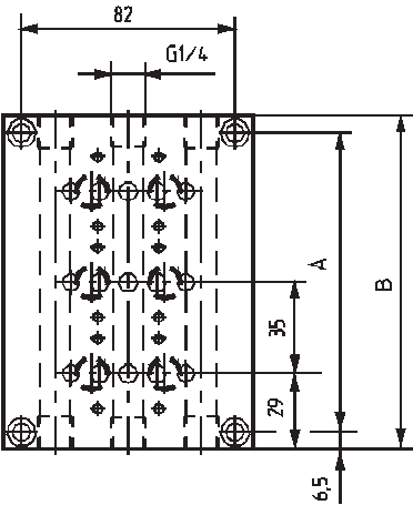
Mehrfachanschlußplatten
