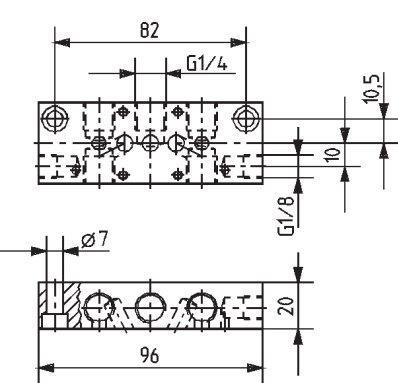
Einzelanschlußplatte
